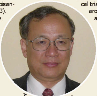
Tohru Fukuyama
